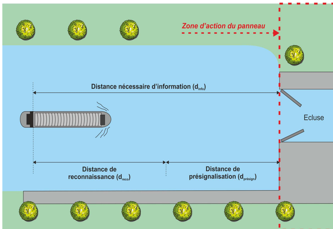
Illustration 20: distance d'information, de reconnaissance, de présignalisation (source : cerema)
