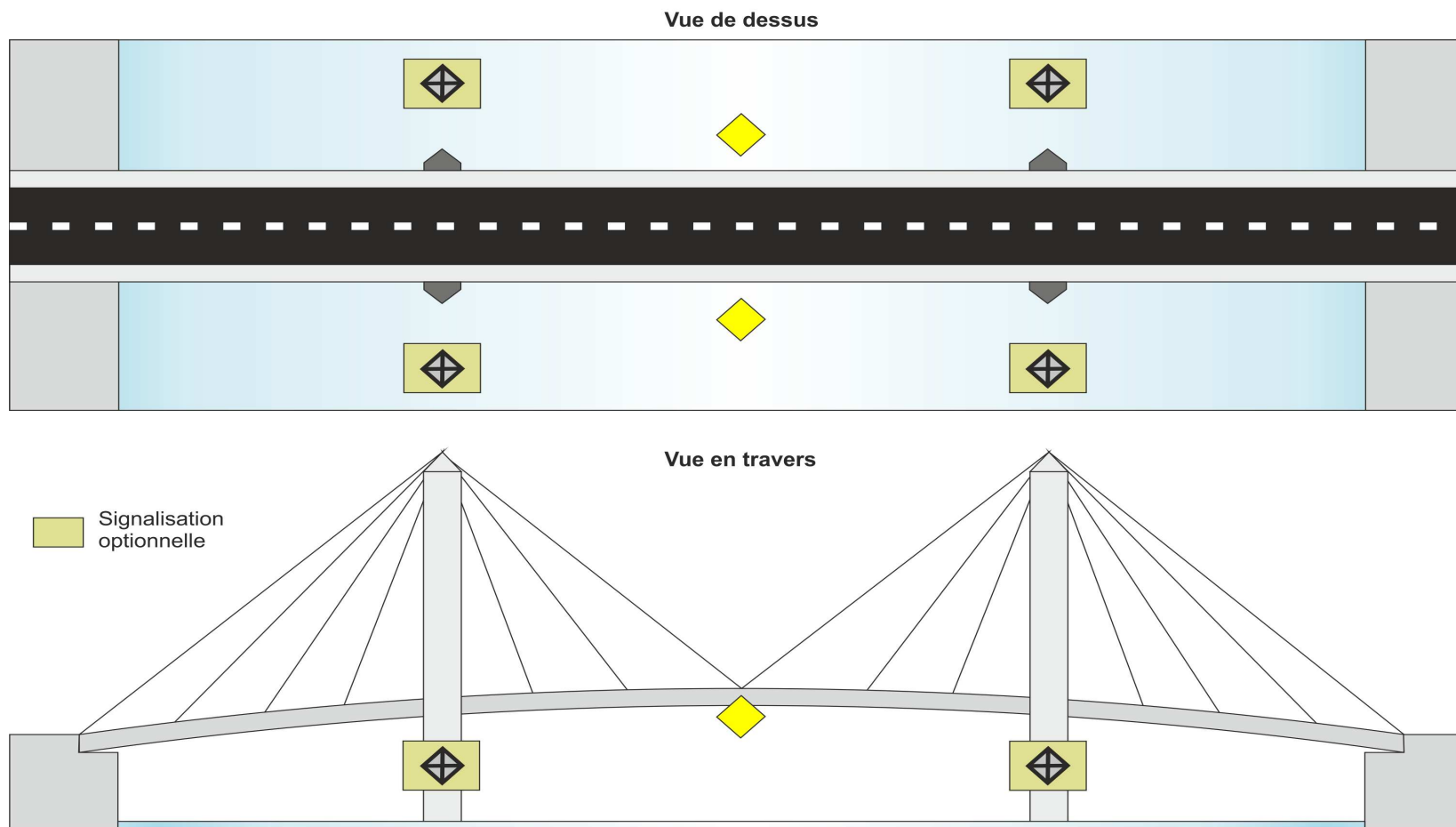
Fiche 4.1 : pont arche unique double sens sans nécessité de préciser le rectangle de navigation
